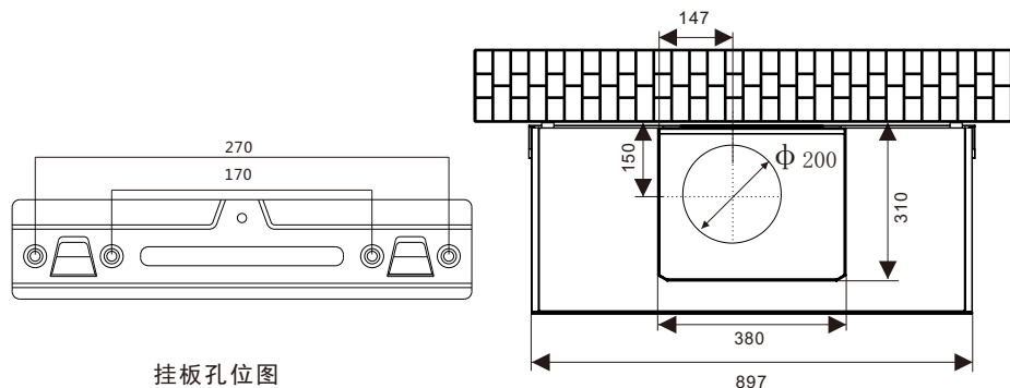
吊顶出风管开孔示意图
